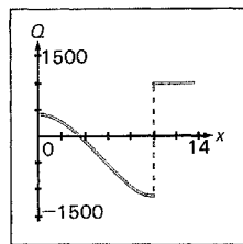
Graph von Q(x)
