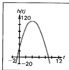
Graph von h(t)
