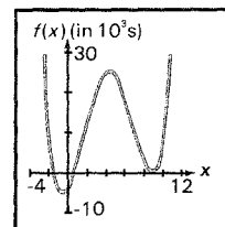
Graph von f(x)
