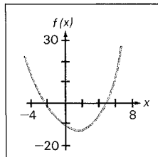
Graph von f(x)
